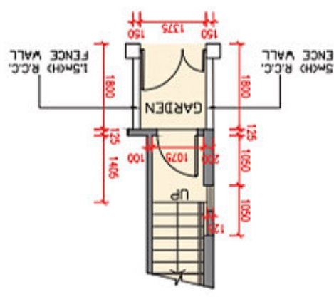
G/F 地下
