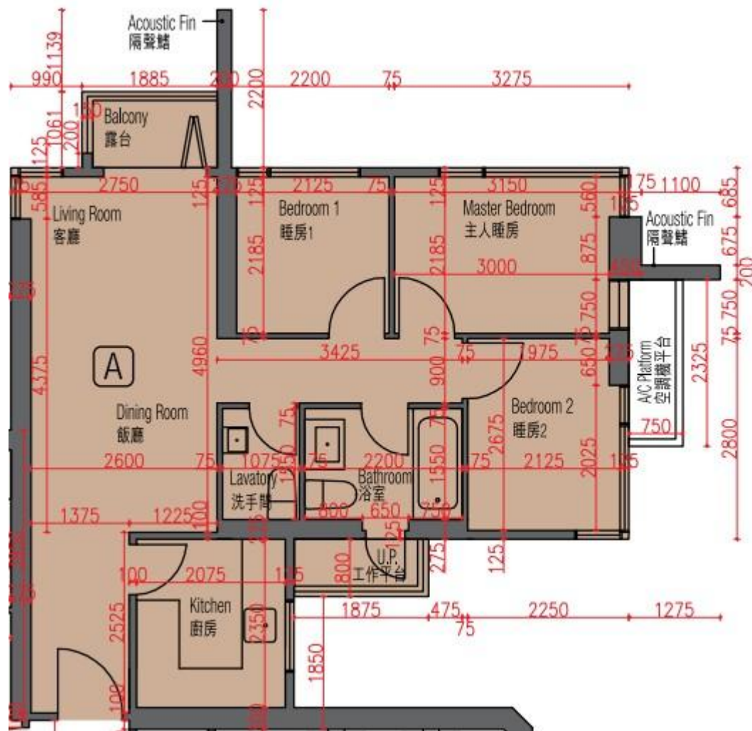
PART PLAN AT 31/F ONLY 局部平面圖 只位於三十一樓
